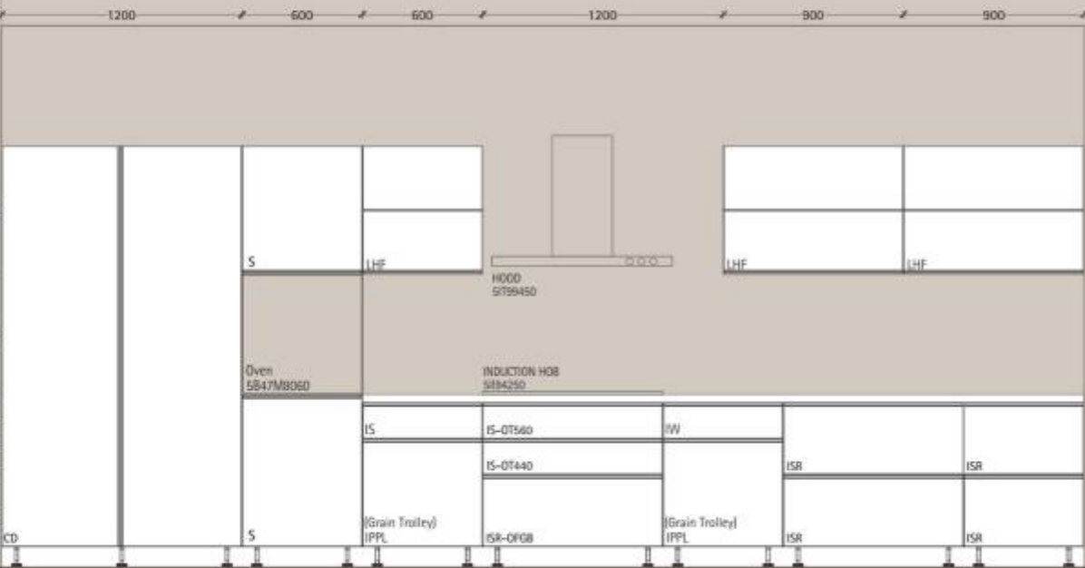
Elevation A
