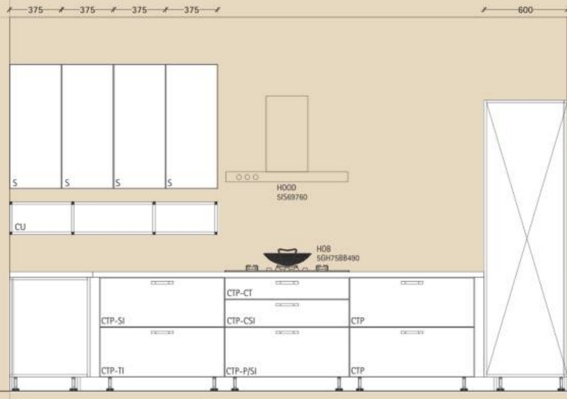
Elevation A
