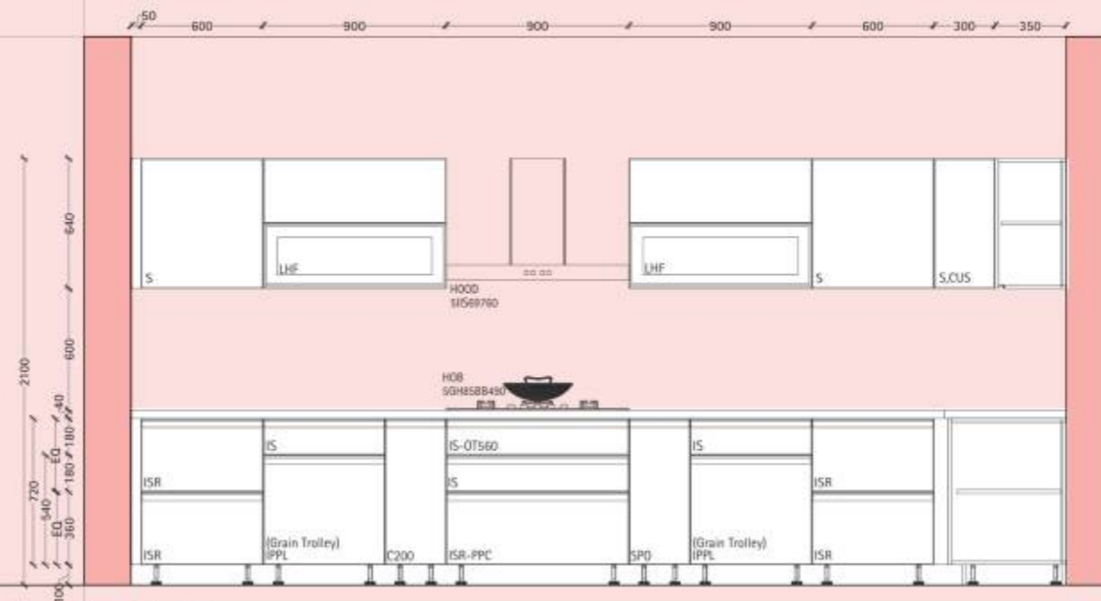
Elevation A
