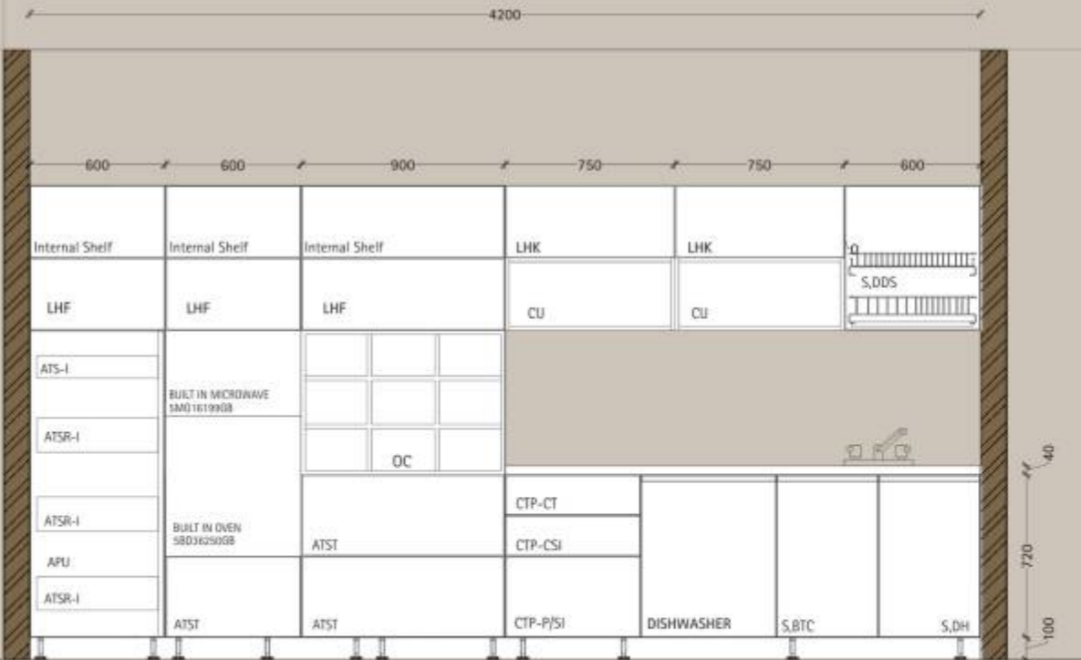
Elevation A
