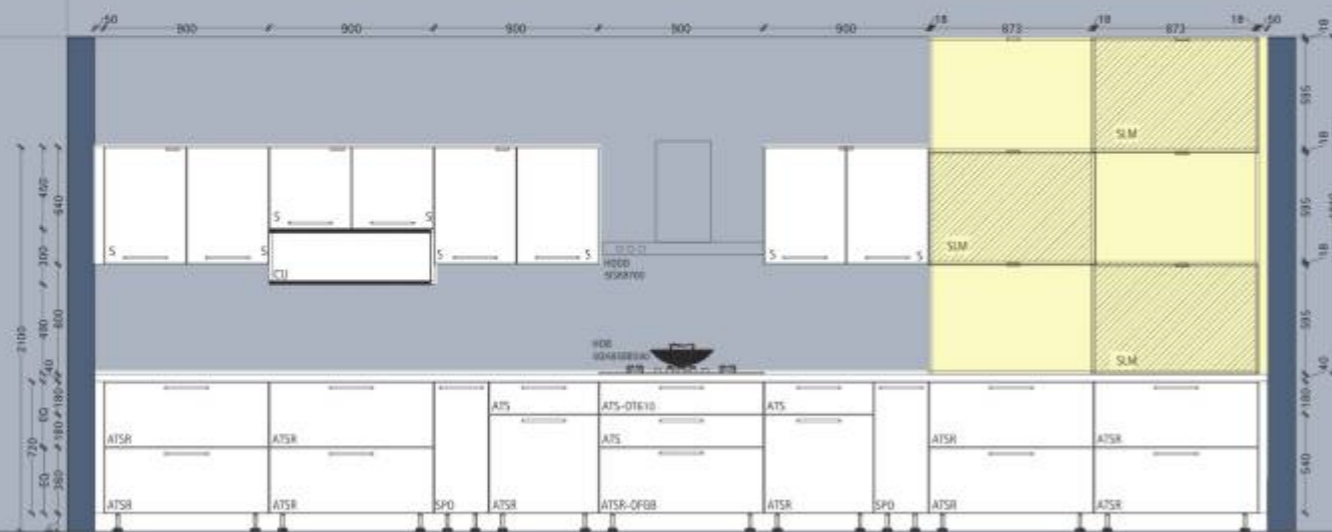
Elevation A
