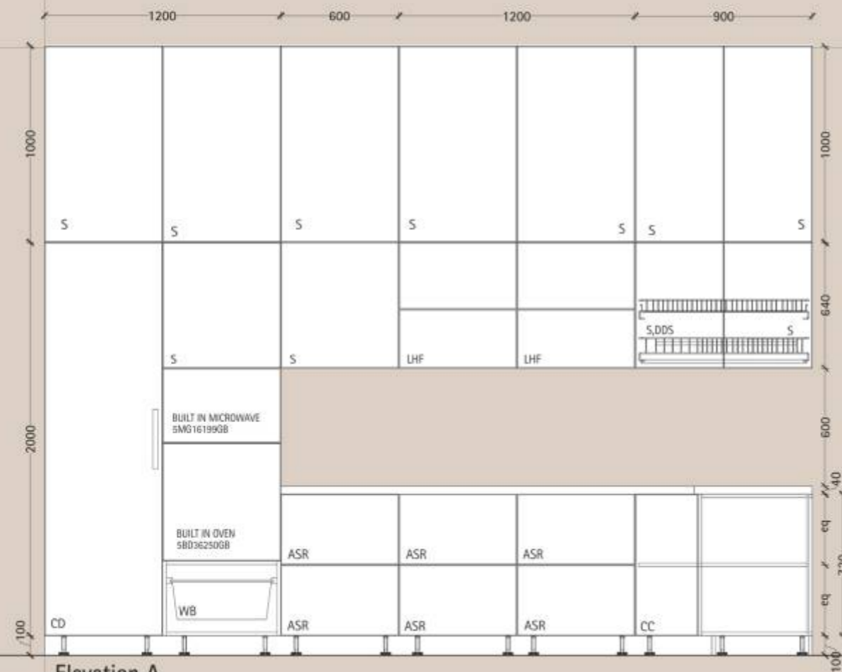
Elevation A
