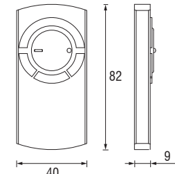
Telecomando IR IR Remote control / IR Fernsteuerung
